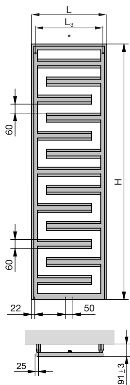
Teplovodná prevádzka: stredové pripojenie
