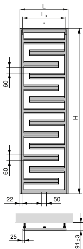
Teplovodná prevádzka: vonkajšie pripojenie
