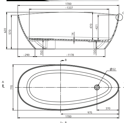
spodná strana vane Atira
